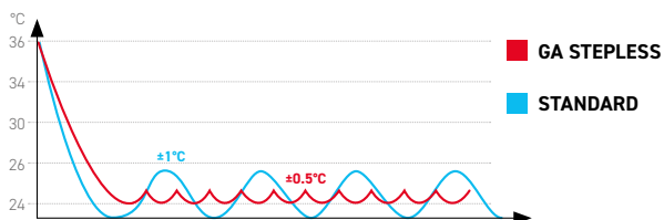
TEMPERATURNI GRAF
